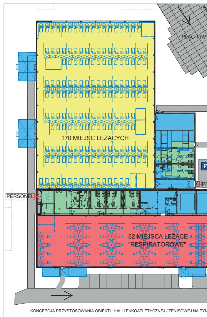
Koncepcja przekształcenia dwóch hal sportowych MOSiR-u przy ul. Sulechowskiej - w szpital tymczasowy dla pacjentów covidowych. W części zaplanowali oddział z łózkami respiratorowymi dla pacjentów wymagających terapii wentylacji
