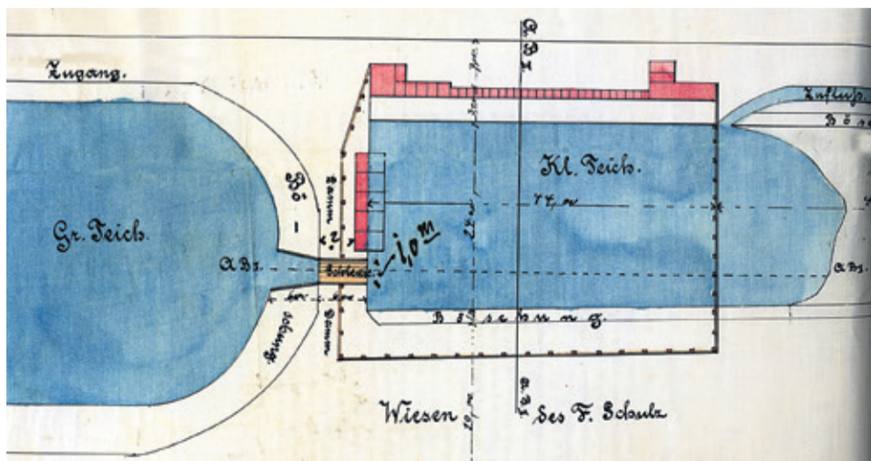
Plan basenu przedstawiony policji budowlanej. Do restauracji trzeba było pójść w lewo, w kierunku dzisiejszej ul. Sulechowskiej. Ze zbiorów Archiwum Państwowego w ZG
