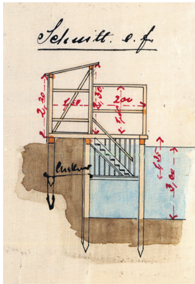
Plan przebieralni wraz z zejściem do wody. Na basenie było pięć takich ekskluzywnych kabin.
