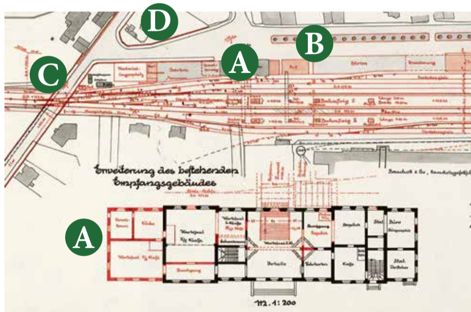
Projekt przebudowy dworca z 1925 r. Czerwoną linią zaznaczono nowe elementy, w tym torowiska. Na dole rysunku plan dworca obrócony o 180 stopni w stosunku do ul. Dworcowej. A - dworzec, B - ul. Sulechowska, C - ul. Dworcowa, D - pl. Kolejarska.
